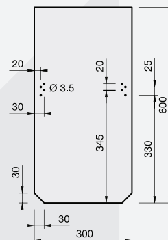
ŠABLONA OBDÉLNÍK SE ZKOSENÝMI ROHY 30×60 cm
