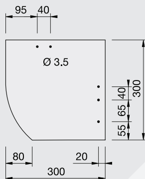
ŠABLONA ČTVEREC S OBLOUKEM 30×30 cm (německé krytí)
